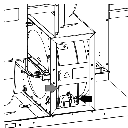
Rys. 3 Pasek napędowy wymiennika obrotowego
