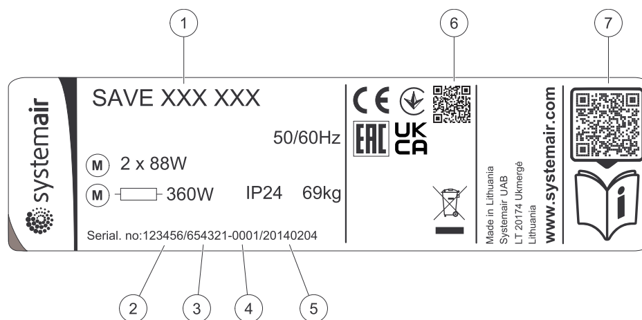
Rys. 1 Tabliczka znamionowa
